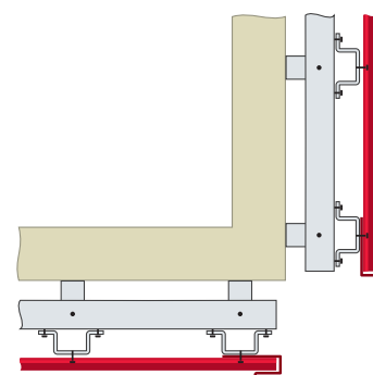
сложная планка внешнего угла
